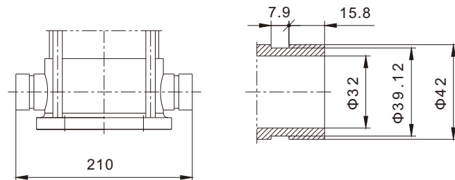
进出口卡口联接尺寸(可选)
