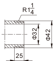
进出口螺纹联接尺寸(可选)
