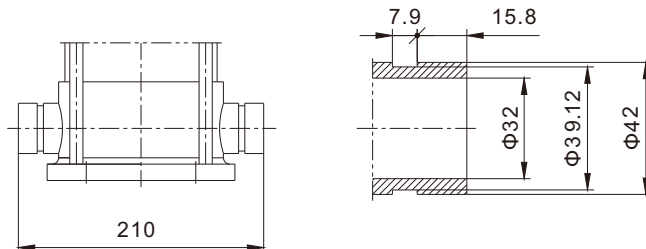
进出口卡口联接尺寸(可选)
