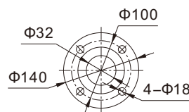
进出口法兰尺寸(标准配置) GB/T17241.6-2008 PN2.5MPa
