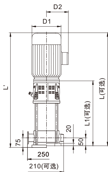
进出口法兰尺寸(标准配置) GB/T17241.6-2008 PN2.5MPa
