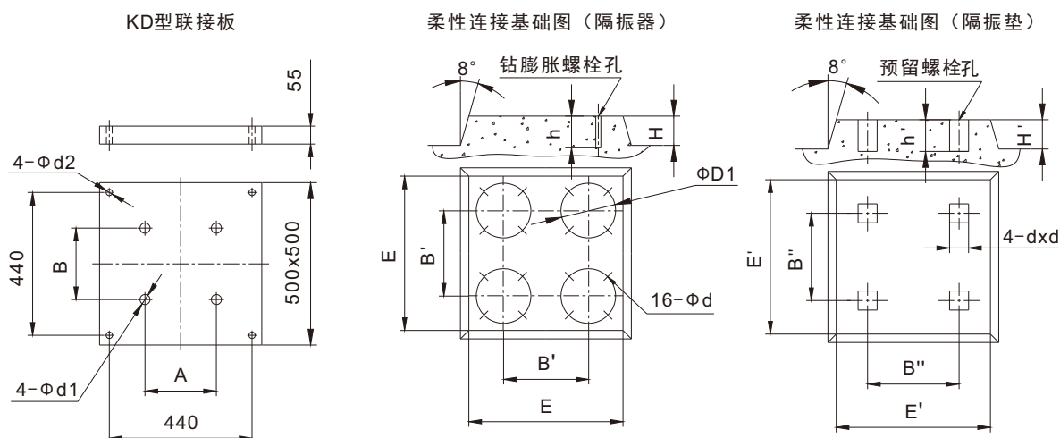
柔性安装基础尺寸图
