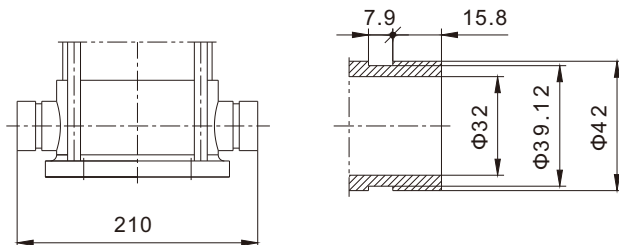
进出口卡口联接尺寸(可选)
