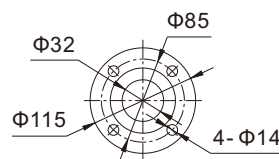
进出口法兰尺寸(标准配置) GB/T17241.6-2008 PN2.5MPa
