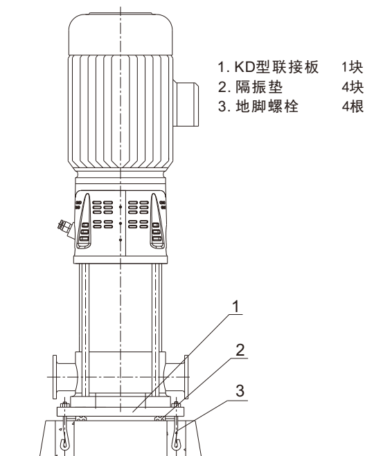
柔性连接（隔振垫）
