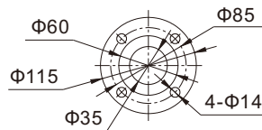
进出口法兰尺寸(标准配置) GB/T17241.6-2008 PN2.5MPa
