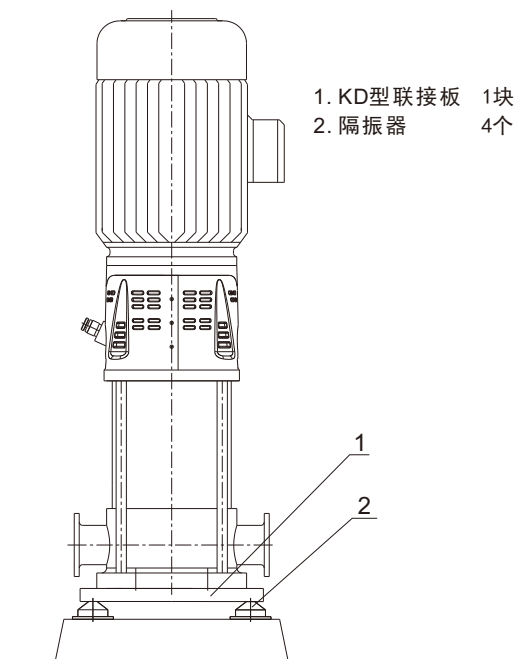
柔性连接（隔振器）
