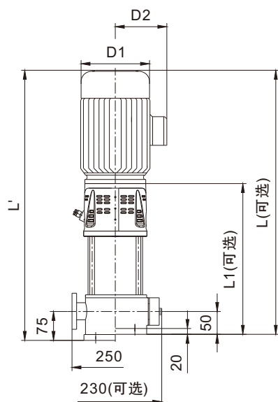
进出口法兰尺寸(标准配置) GB/T17241.6-2008 PN2.5MPa
