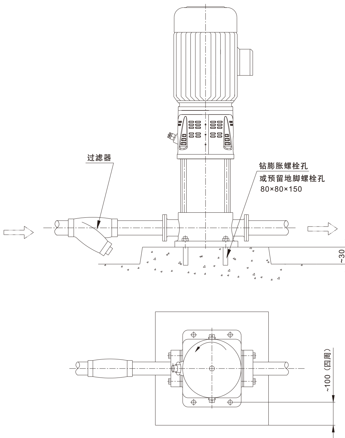
KQDP、KQDQ 安装图
