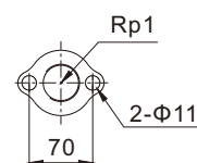
附配对进出口椭圆法兰联接尺寸 (可选 PN1.6MPa)
