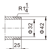
进出口螺纹联接尺寸(可选)
